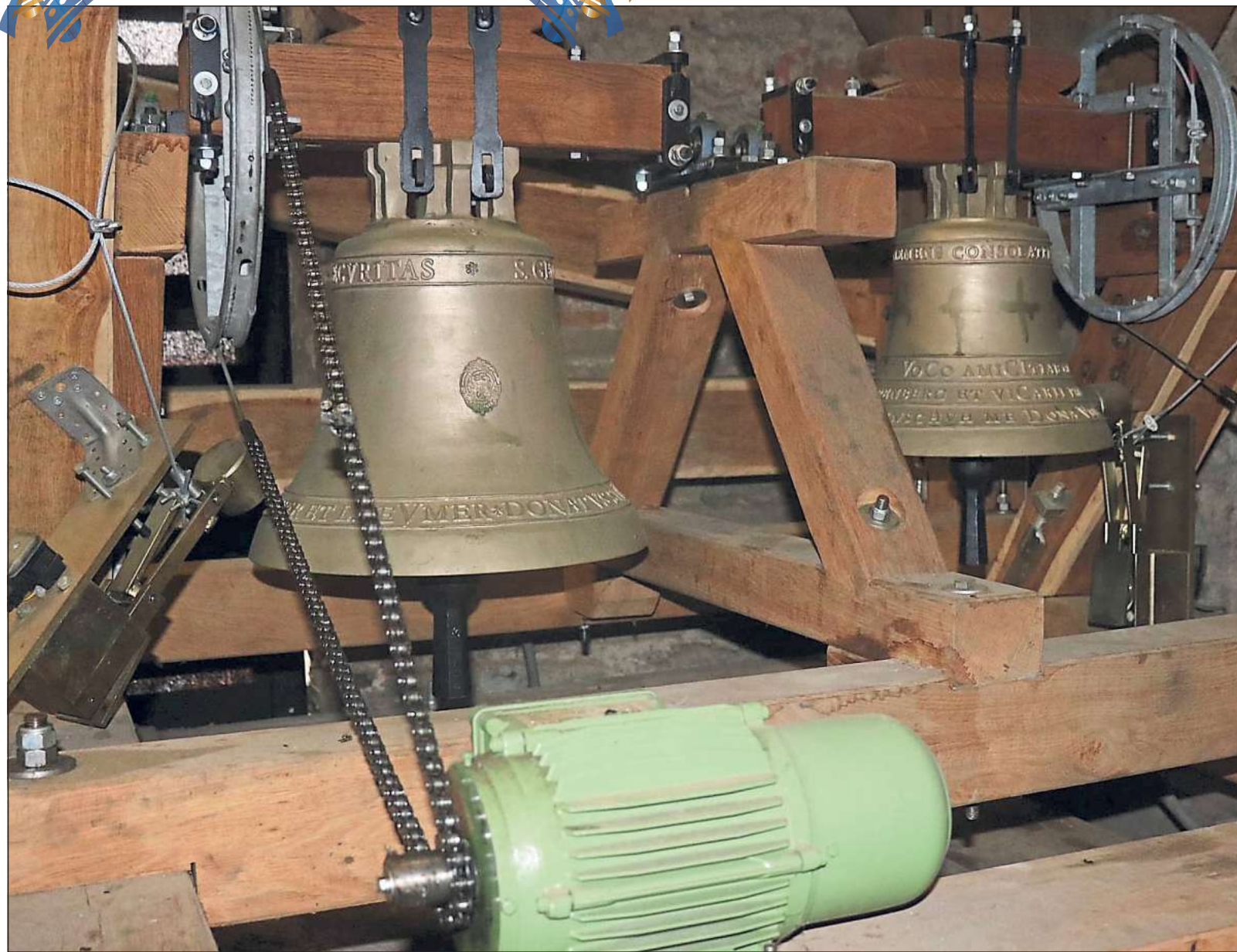
Bronzene Klangkörper: Zwei der Glocken des 15-teiligen Glockenspiels der St.-Stephanus-Kirche in Beckum. An den beiden Außenseiten sind die Magnethammer zu erkennen, mit denen die Töne geschlagen werden. Fotos: Niemeyer
